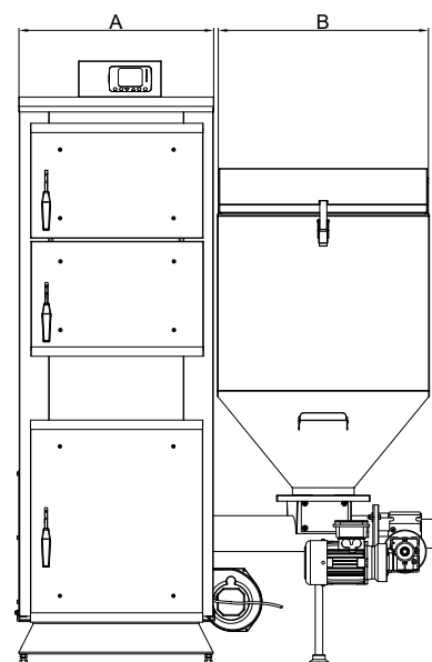
Kocioł z wyprowadzeniem spalin poprzez czopuch do góry
